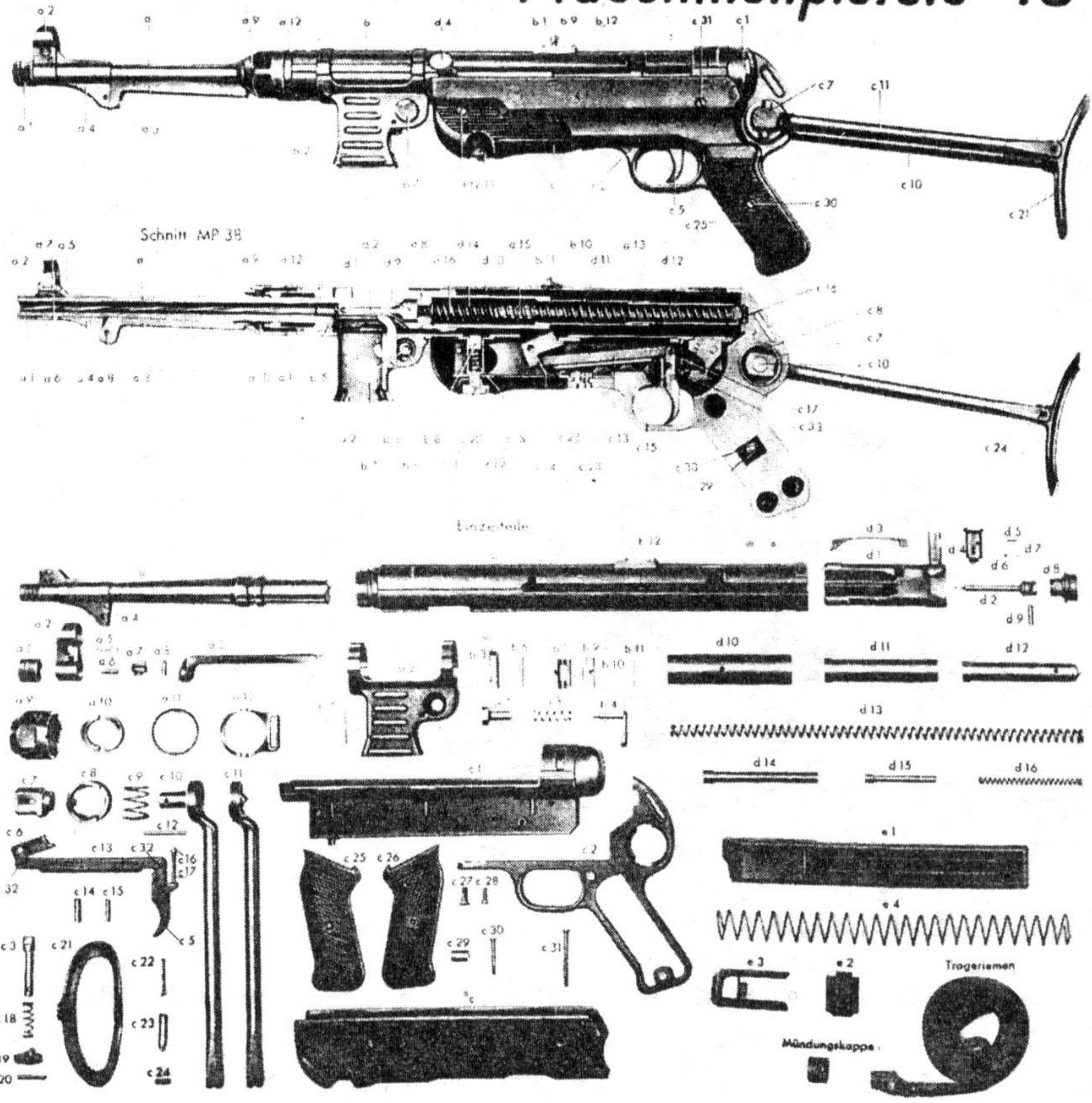
Армейский плакат для изучения материальной части MP.40. Такие плакаты висели в казармах и на полигонах Вермахта.
