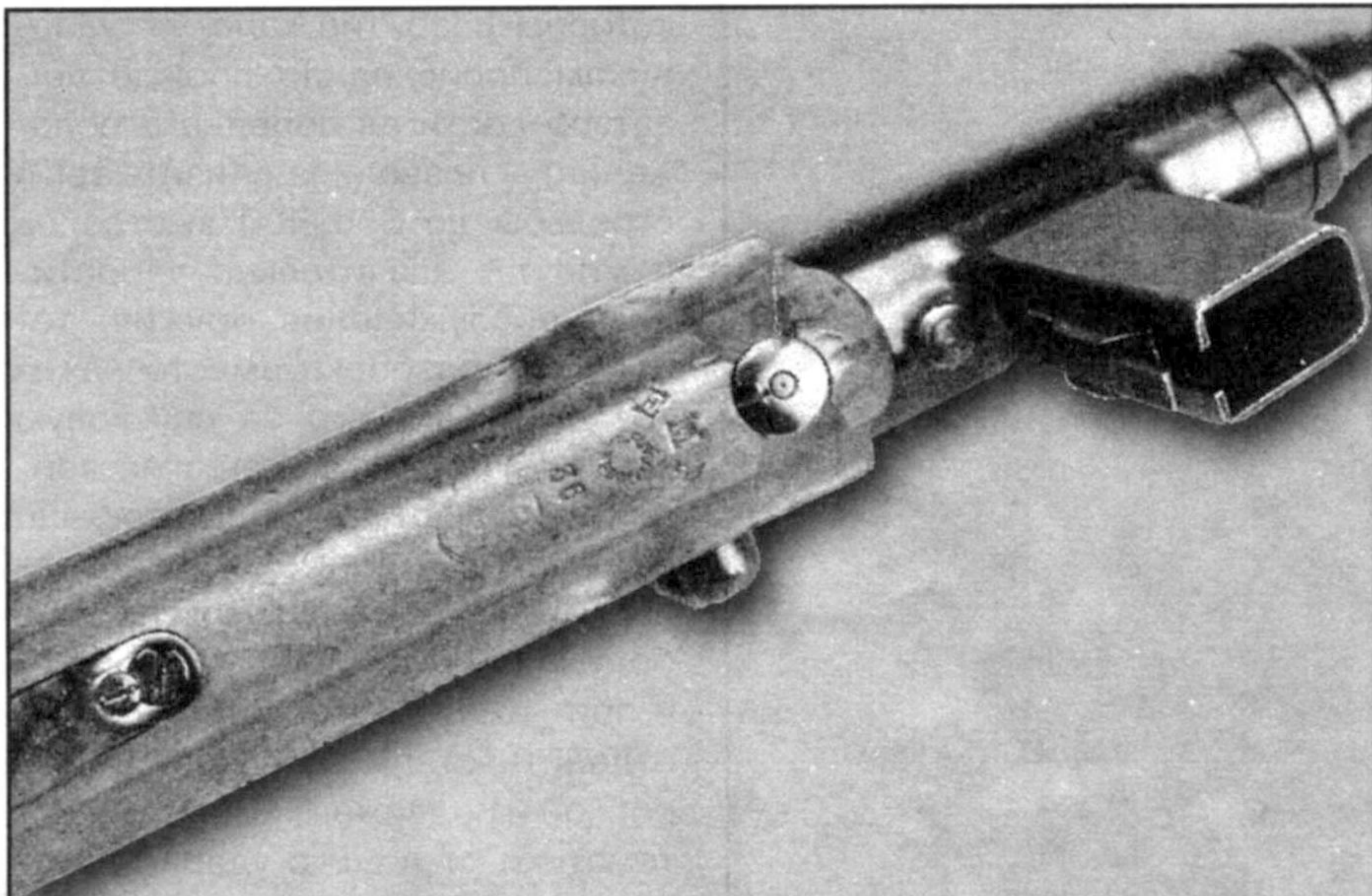
Вид снизу на цевье и затворную коробку ERMA 36. В передней части цевья имеется стопорный болт, обеспечивающий быструю и удобную разборку и сборку оружия. Отвод горловины магазина влево, видимо, должен был облегчить зарядание.
